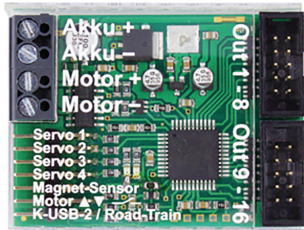
Auflieger-Lichtmodule LM-IR-16-4/LM-BT-16-4 von BEIER-Electronic
