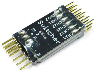
Kanalerweiterungsmodul Switcher von Pistenking
