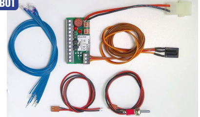
Auflieger-Lichtanlage MFL-A von WEDIC0models
