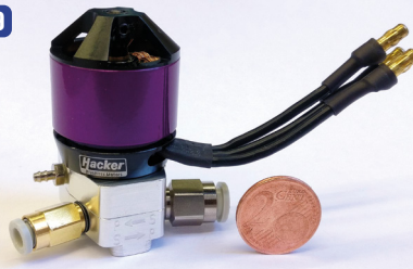
Mikro-Hydraulikpumpe von Braeker
